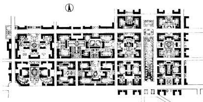
图10 长春第一汽车制造厂居住区中式住宅街坊总平面图
